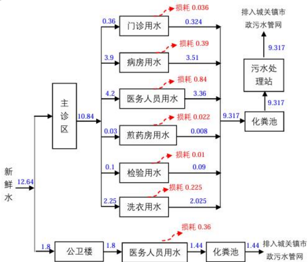
图 2-1 水平衡图 (m³/d)
