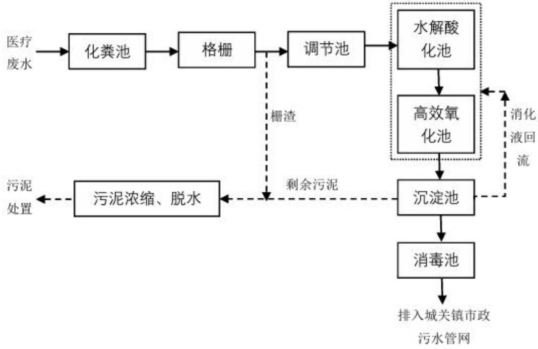
图 4-1 本项目污水处理工艺流程图
