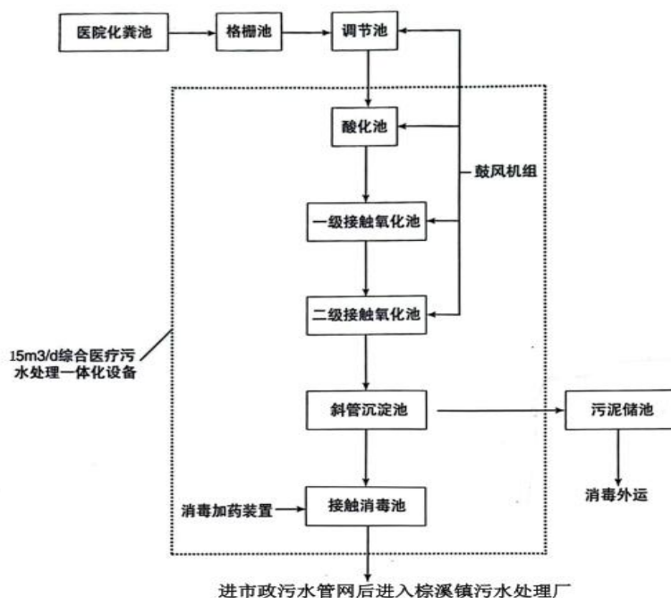
图 4-1 本项目废水处理工艺流程图
