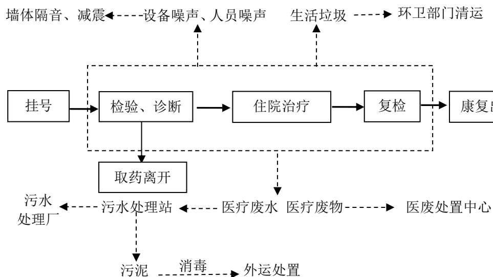
图 2-2 项目运营期工艺流程图
