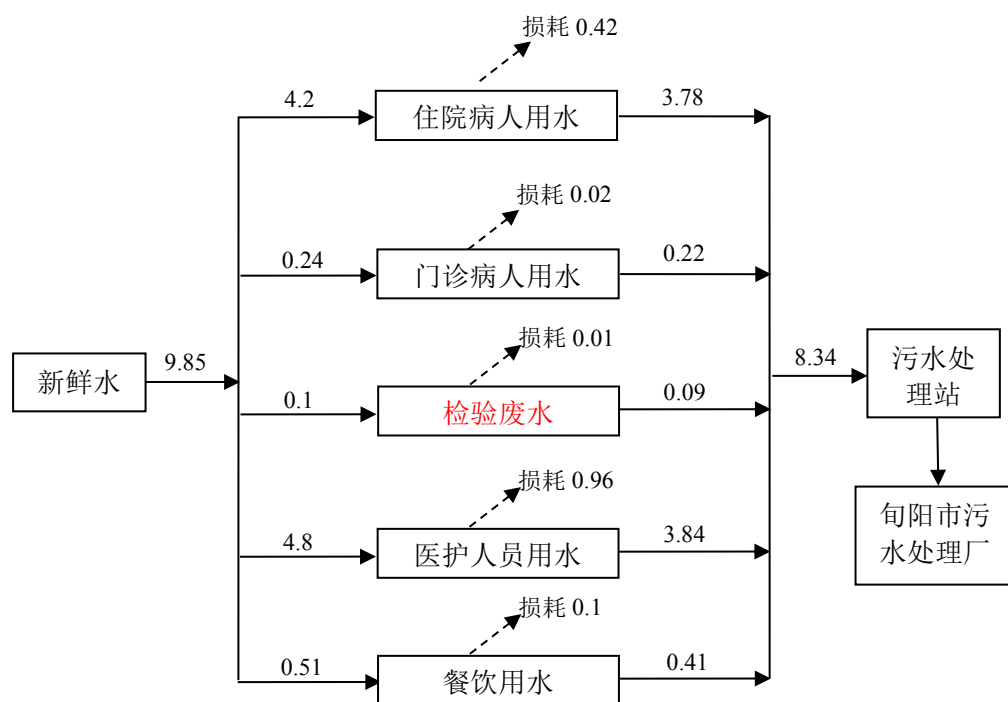
图 2-1 拟建项目水平衡图 (m³/d)
