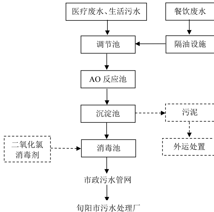
图 4-1 污水处理工艺流程图
