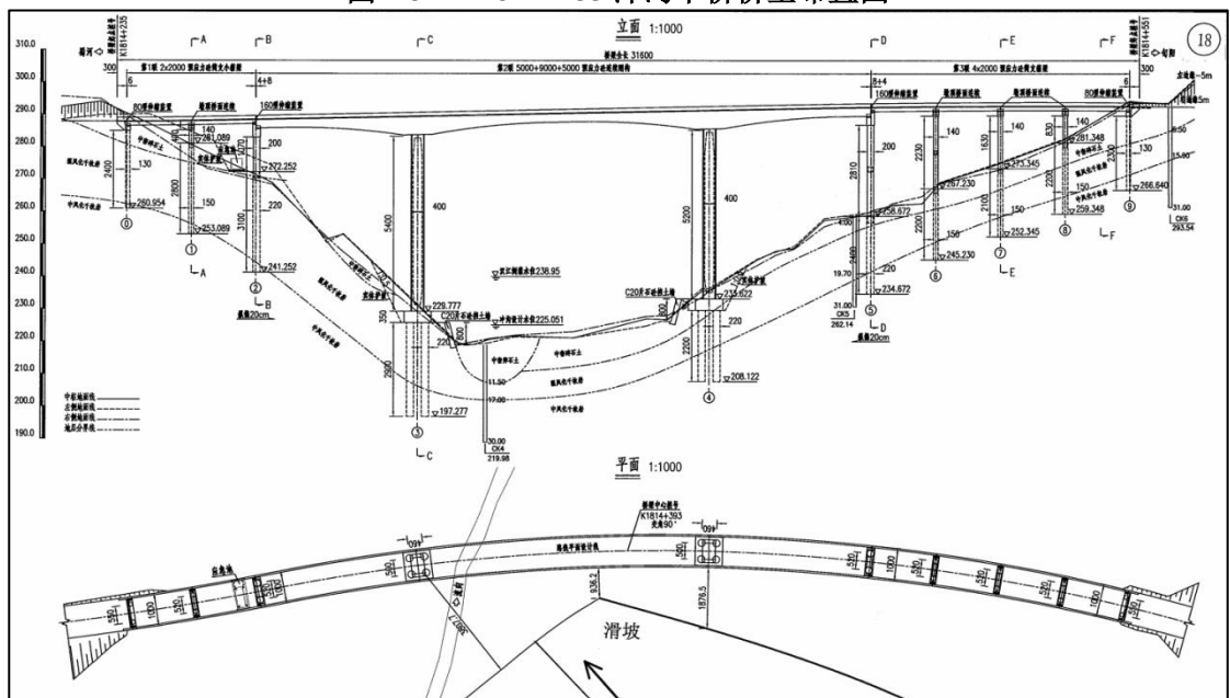
图 2-4 K1814+393 唱郎沟大桥桥型布置图
