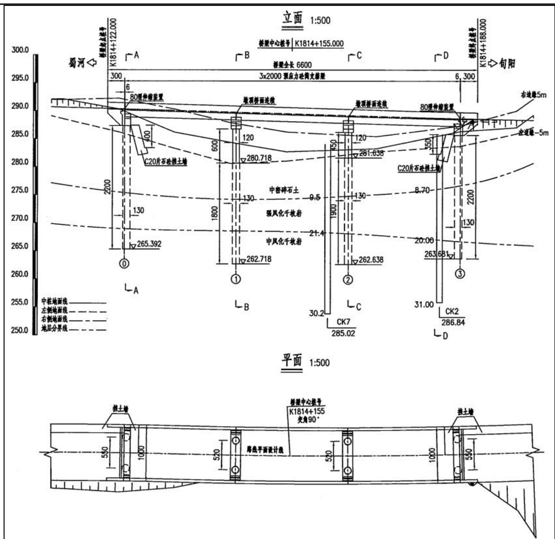
图 2-3 K1814+155 冲沟中桥桥型布置图
