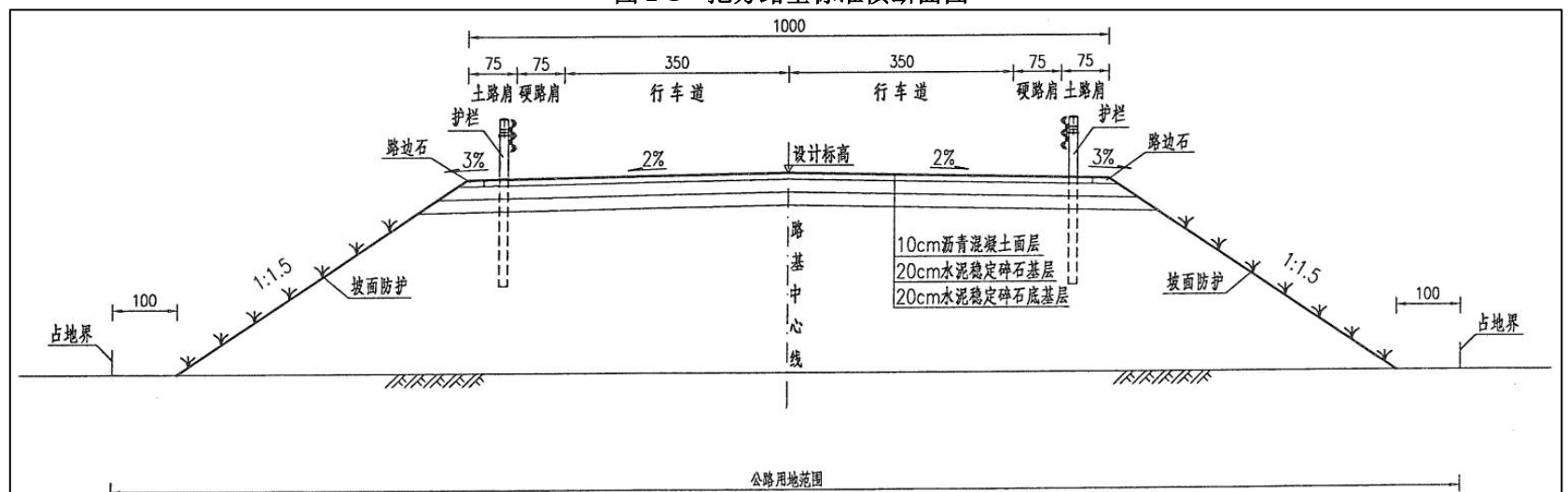
图 2-2 填方路基标准横断面图
