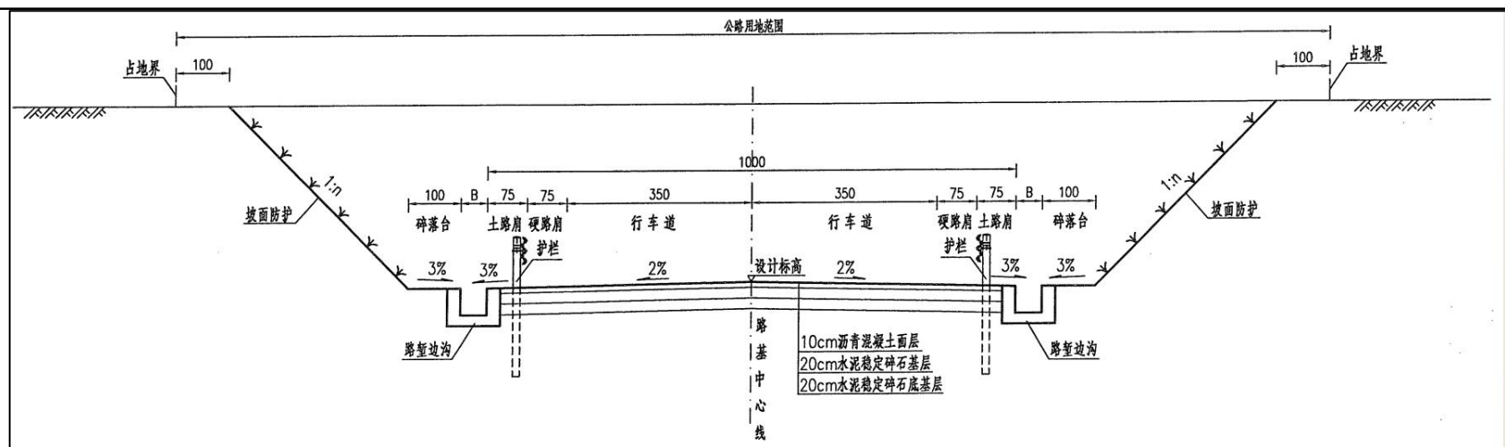
图 2-1 挖方路基标准横断面图
