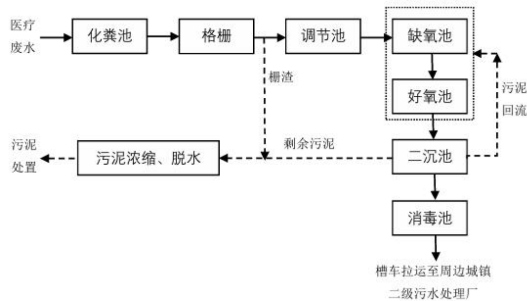
图 4-1 本项目污水处理工艺流程图
