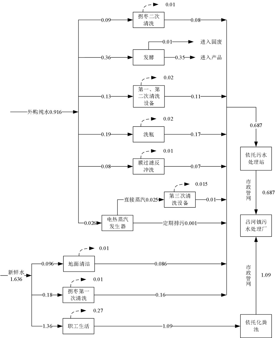
图 2-1 项目水平衡图 m 3 /d
