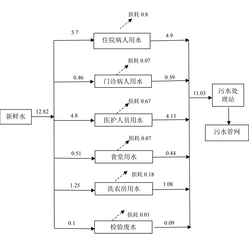
图 2-1 拟建项目水平衡图（m³/d）
