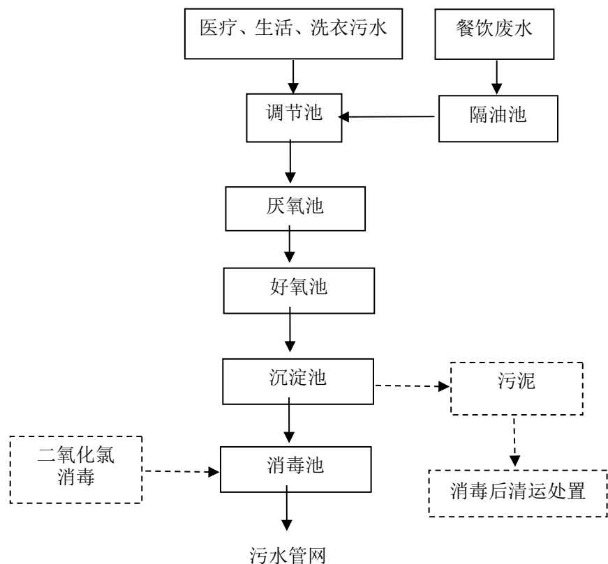
图 4-1 污水处理工艺流程图
