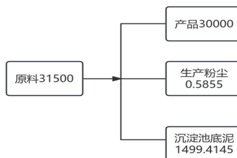
图2.1项目物料平衡图（单位：t/a）
