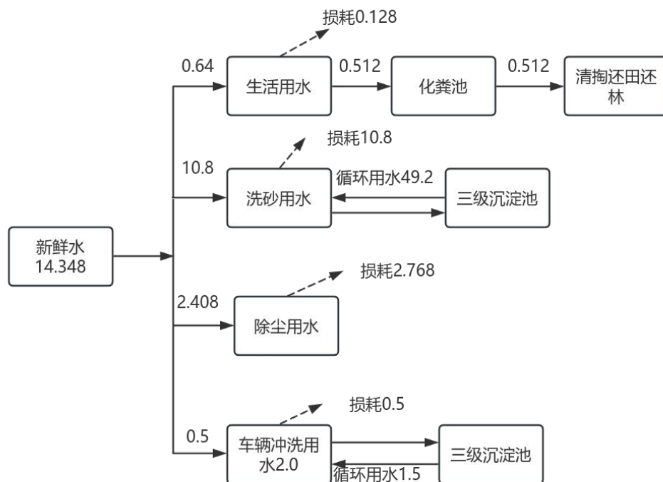
图2.2水平衡示意图 (单位: m 3 /d)
