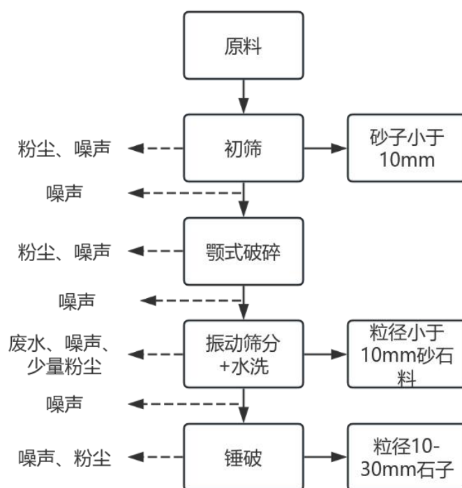
图 2.4 生产工艺流程及产污环节
