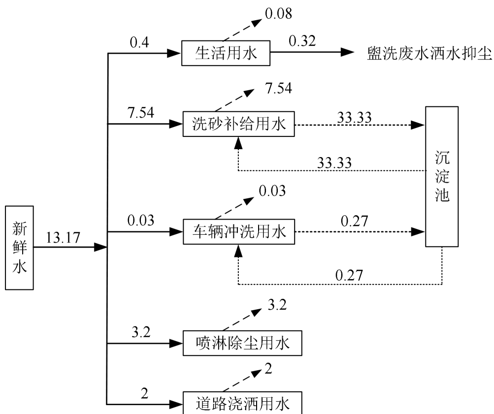
图2 本项目水平衡图 （单位：m 3 /d）
