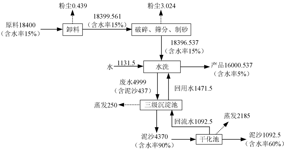
图 2-1 本项目物料平衡图 （单位：t/a）
