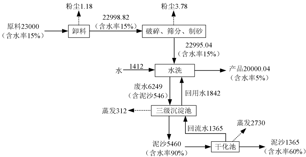
图 2-1 本项目物料平衡图 （单位：t/a）
