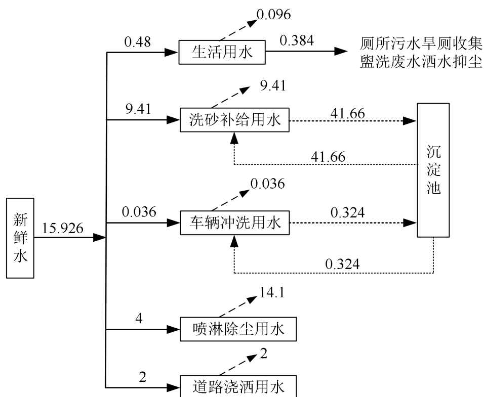
图2-2 本项目水平衡图 (单位: \text{m}^3/\text{d} )
