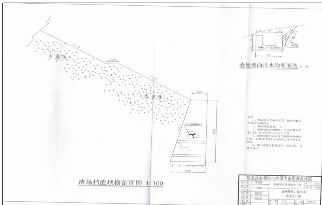
图2-5 渣场拦渣坝、戽台及排水沟设计图
