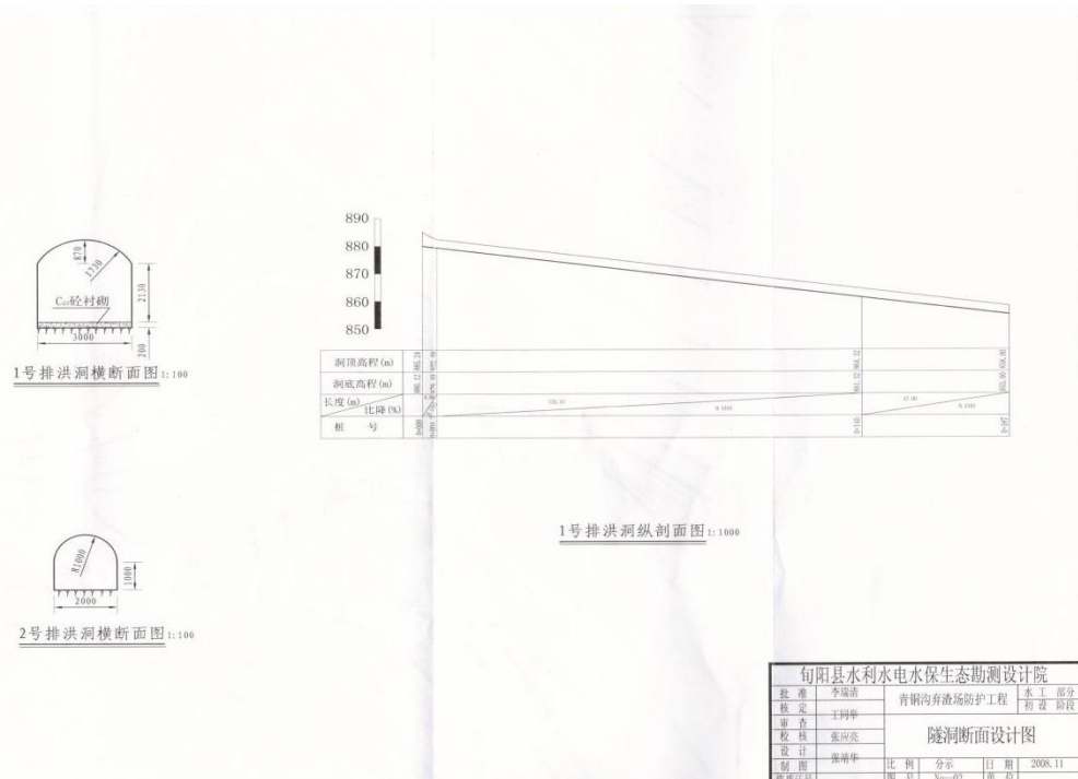
图 2-1 1、2 号隧洞设计断面设计图
