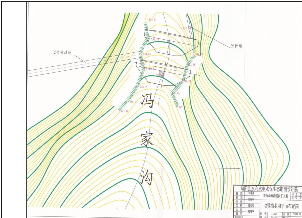
图 2-3 2 号挡水坝平面布置图
